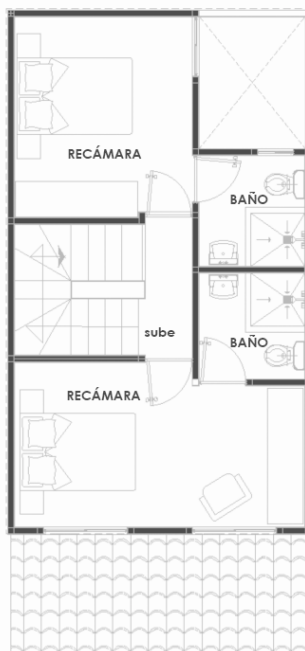
PLANTA ALTA
